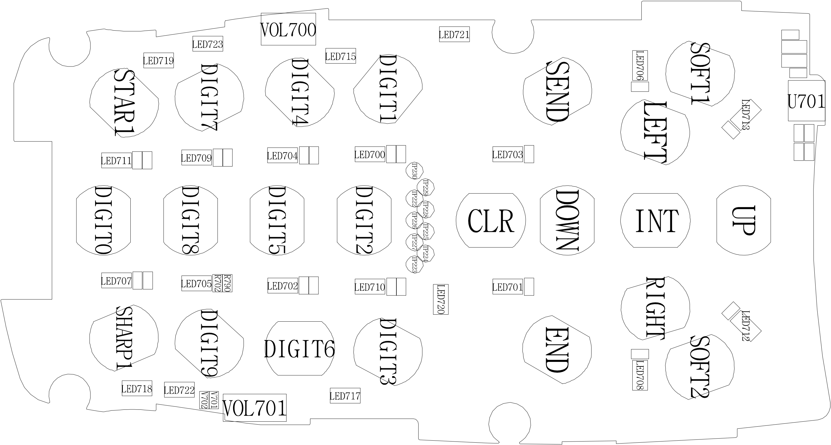
6-2. PCB Bottom Diagram
