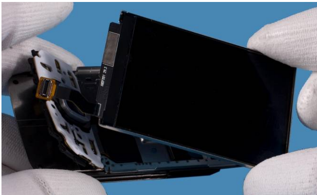
39) Remove the LCD.
