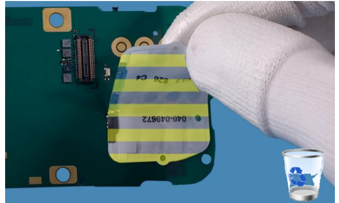
20) Remove the DOMESHEET .
