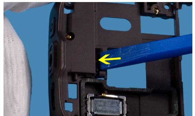
30) Press out the AV CONNECTOR .
