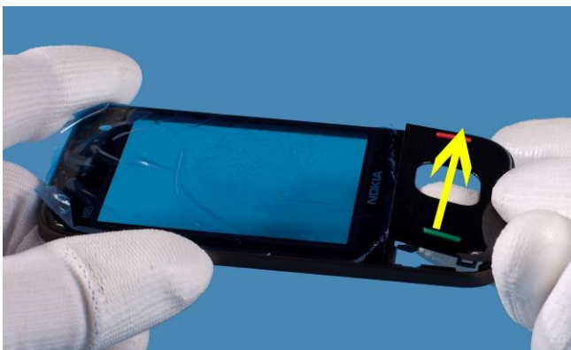
35) Press out the S60 KEYMAT .
