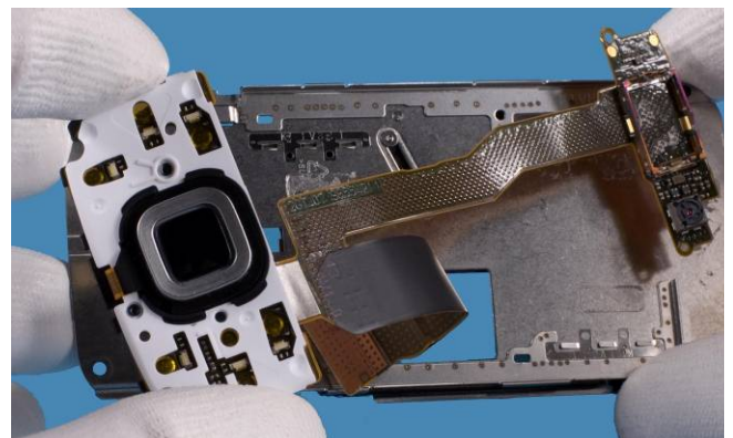
42) Remove the UI-FPC ASSY .
