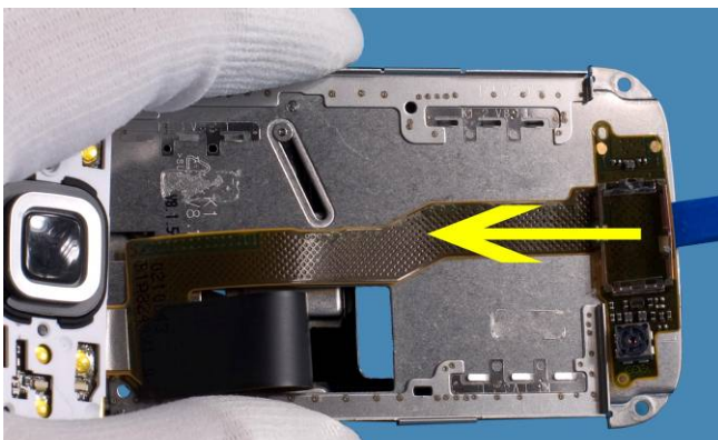
41) Detach the UI-FPC ASSY .
