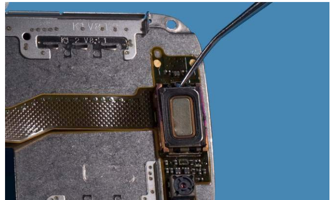
40) Remove the EARPIECE .
