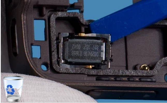
31) Remove the IHF SPEAKER .
