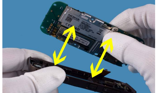
14) Remove the PWB .
